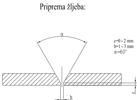
Skica žljeba
